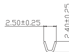
SEC:A-A
